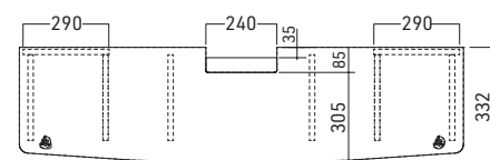
上面
