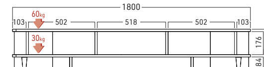
前面
