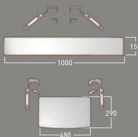
HDDホルダー WS-HLD100 ●質量/0.2kg ●耐荷重/2kg 結束ベルト付属
